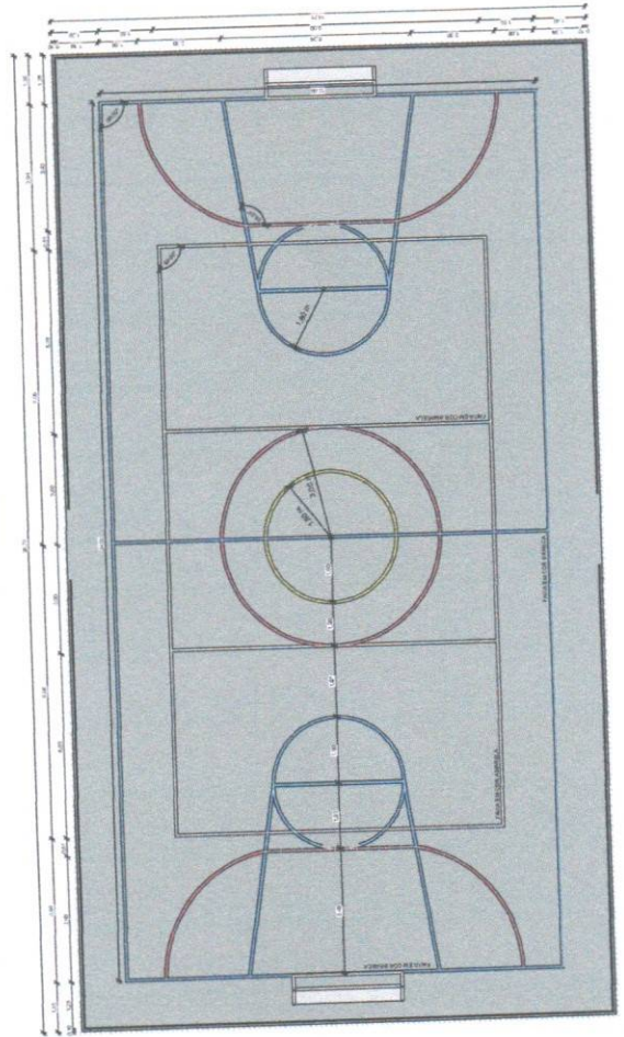
2 - PINTURA DE PISO DA QUADRA - FAXAS (ESCALA 1:20)
