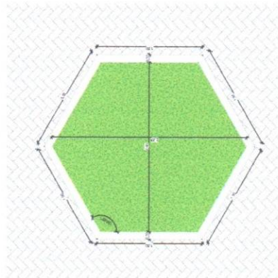
4 - DETALHE DE CANTEIRO HEXAGONAL ESCALA 1:5
