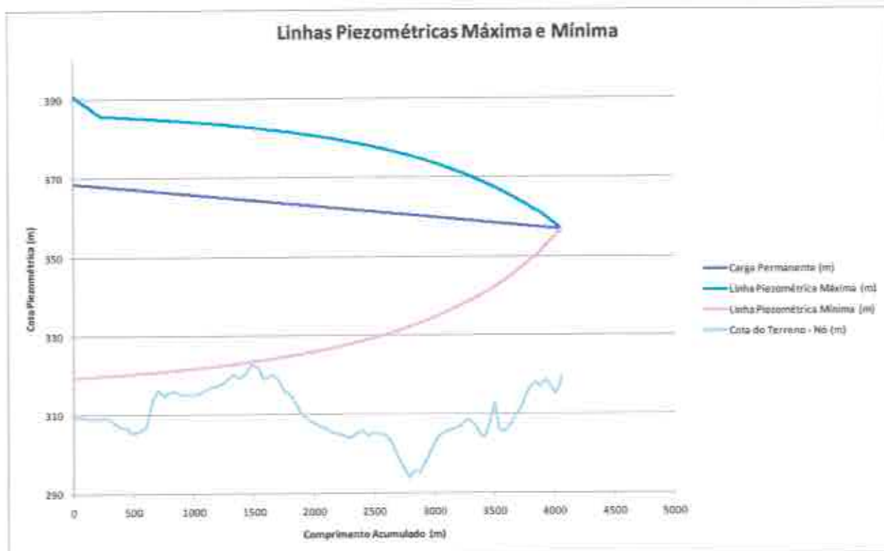
Figura 4.1 – Gráfico de Linhas Piezométricas Máxima e Mínima para a adutora de água bruta de Torres
